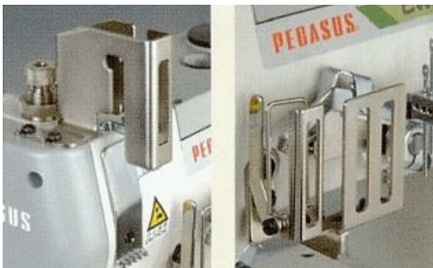
Традиционна система за опън на конците с предпазители за оператора.
